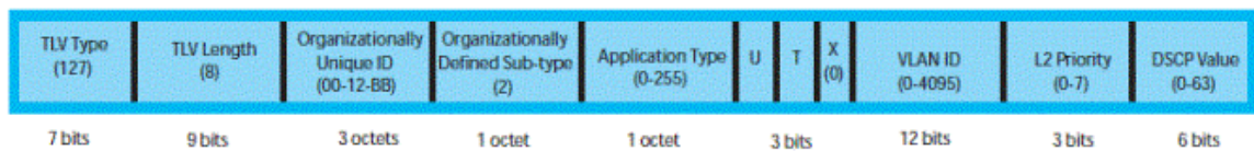
Figure 24. LLDP-MED Policies TLV
